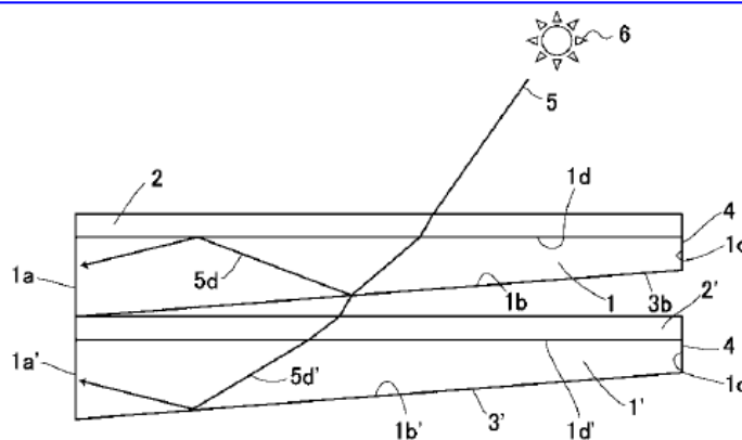
【図1】本発明に係る実施例2の太陽光集光器を示す断面説明図
