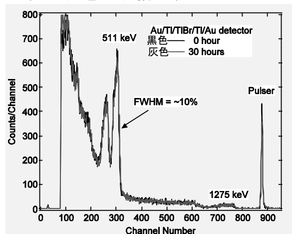
【図2】Au/Tl/TlBr/Tl/Au放射線検出器で測定した 22 Naスペクトル図 連絡先
