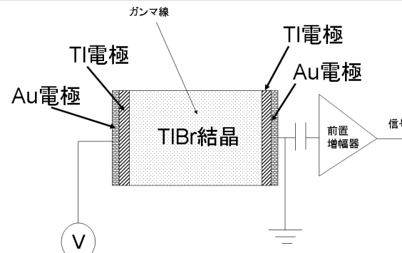
【図1】Auで覆ったTl電極を付けた本発明に係る臭化タリウム放射線検出器を示す構造模式図
