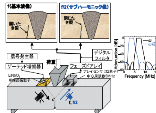
図 サブハーモニック超音波フェーズドアレイの原理と実験方法
