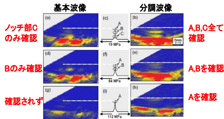
図 SUS316Lにおける荷重依存性
