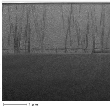
再成長AIN膜 熱処理AIN膜 サファイア基板
