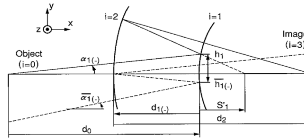
図1. 本発明で取り扱う2面反射結像系を示す図
