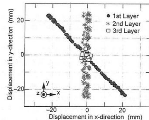
図3 モデル免震装置振動時のリサーチ図形
