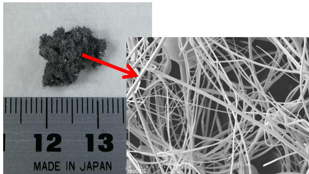
図1. 本発明により作製された金属ガラスナノファイバー
