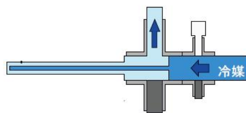
クライオプローブ模式図
