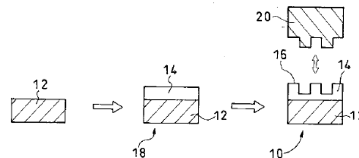
成形体の製造方法の概略を示す図
