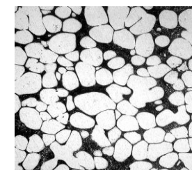
図 足廻り部品・アームの外観写真と金属組織
