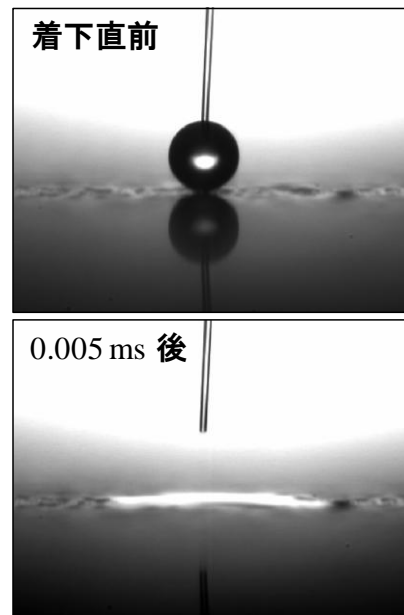
【図2】蛍光灯下での陽極酸化膜への水滴落下後CCD画像: 水滴が高速で濡れ拡がるのが観察できる
